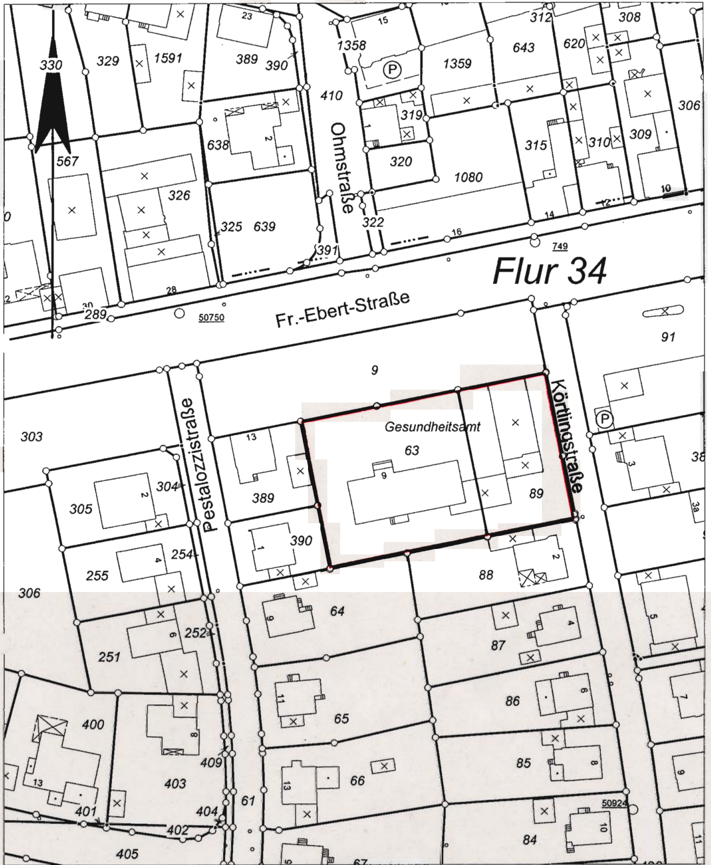
Gemarkung Datteln Flur 34 Maßstab 1:1000
